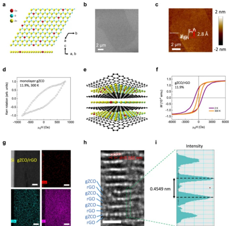
Fig. 1: 2D vdW gZCO.
